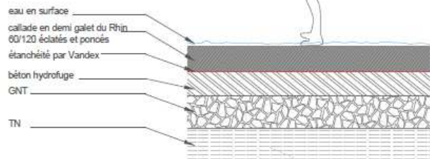
principe d'étanchéité du revêtement 1/20e
