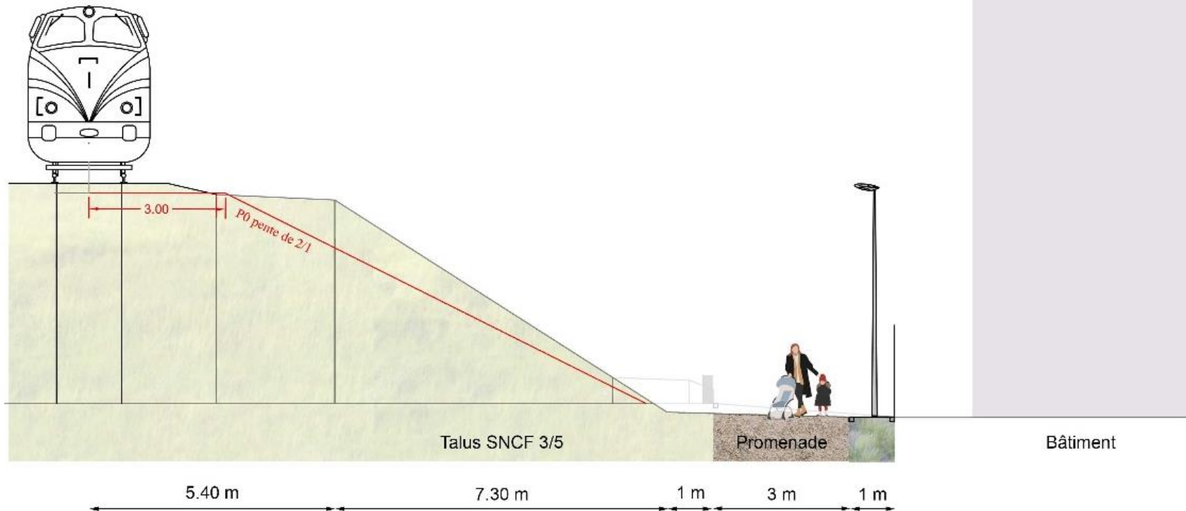
COUPE C1
