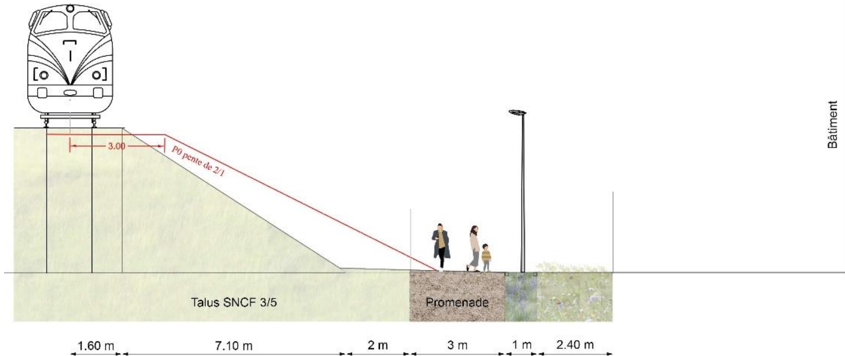
COUPE C2
