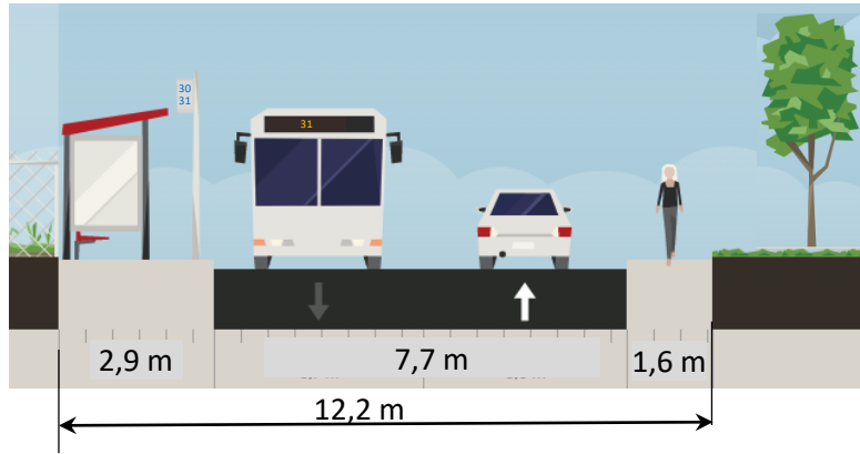
Voirie existante (arrêt Musau)
