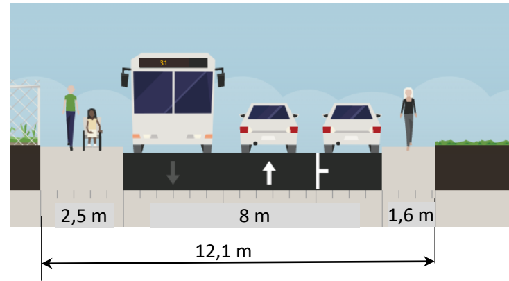
Voirie existante (12 rue de Wattwiller)
