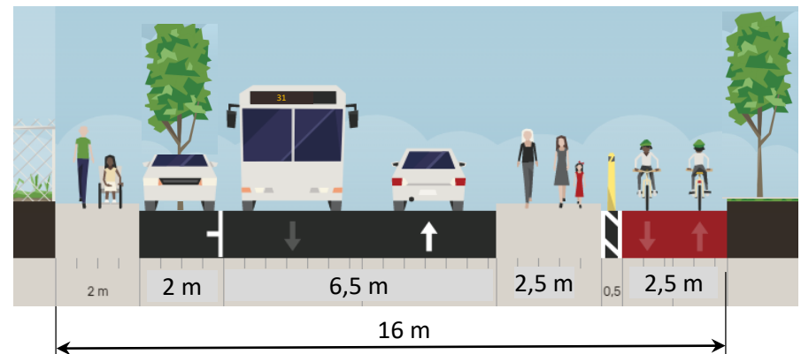
Voirie projetée (12 rue de Wattwiller)
