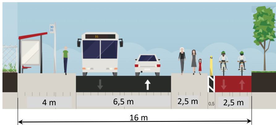
Voirie projetée (arrêt Musau)
